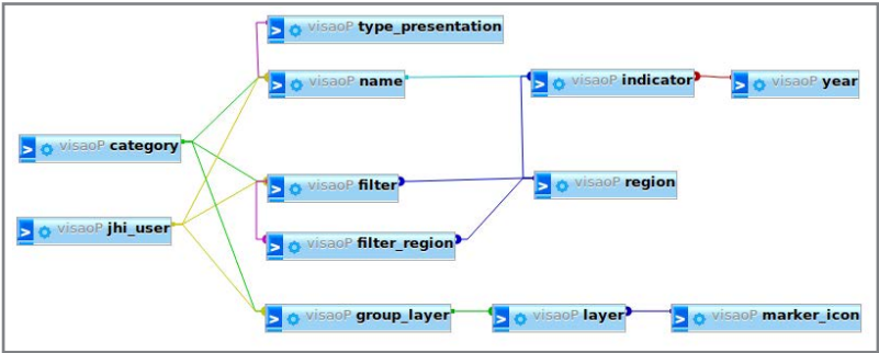
Figura 4.4 - Esquema relacional do banco
